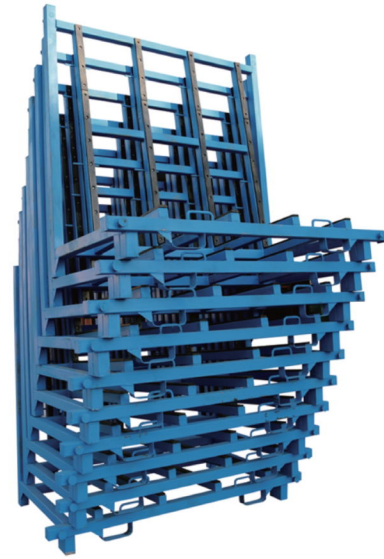
多个叠放、节约场地、方便运输
