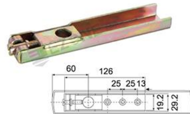
AC-03(下) 枢轴底座: Pivot Bottom Seat
