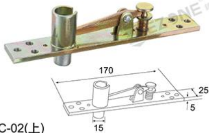
AC-02(上) 上枢轴座: Top Pivot Seat
