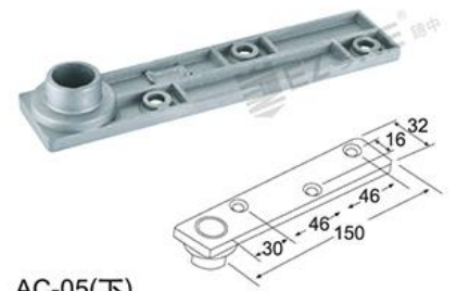
AC-05(下) 枢轴底座: Pivot Bottom Seat
