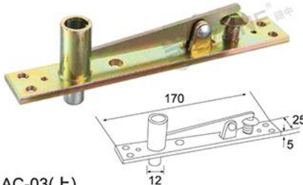
AC-03(上) 上枢轴座: Top Pivot Seat
