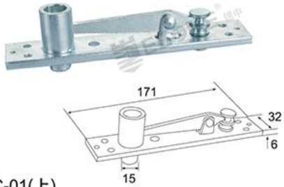
AC-01(上) 上枢轴座: Top Pivot Seat
