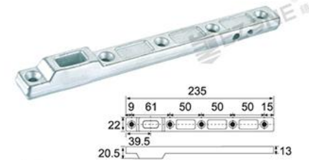
AC-07 中心摇臂: Center Pivoted Arm
