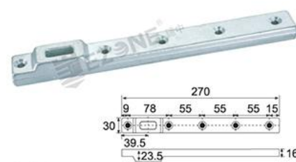
AC-06 中心摇臂: Center Pivoted Arm
