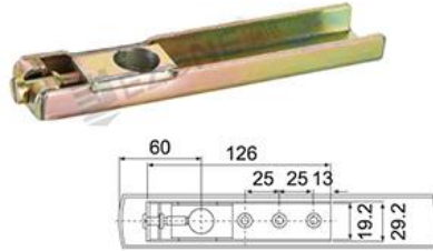
AC-02(下) 枢轴底座: Pivot Bottom Seat
