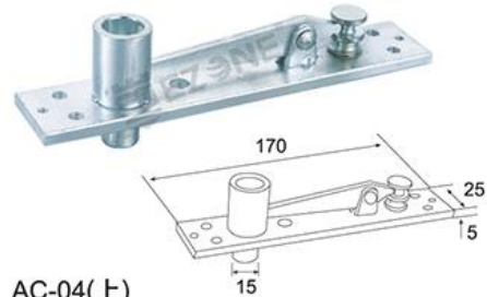
AC-04(上) 上枢轴座: Top Pivot Seat
