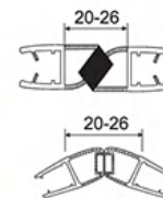
EPV-1421 配装 6/8/10/12mm 玻璃 For:6/8/10/12mm glass
