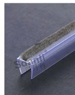
EPV-1427 配装 6/8/10/12mm 玻璃 For:6/8/10/12mm glass
