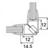
EPV-1428 配装 6/8/10/12mm 玻璃 For:6/8/10/12mm glass
