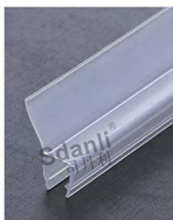
EPV-1425 配装 6/8/10/12mm 玻璃 For:6/8/10/12mm glass
